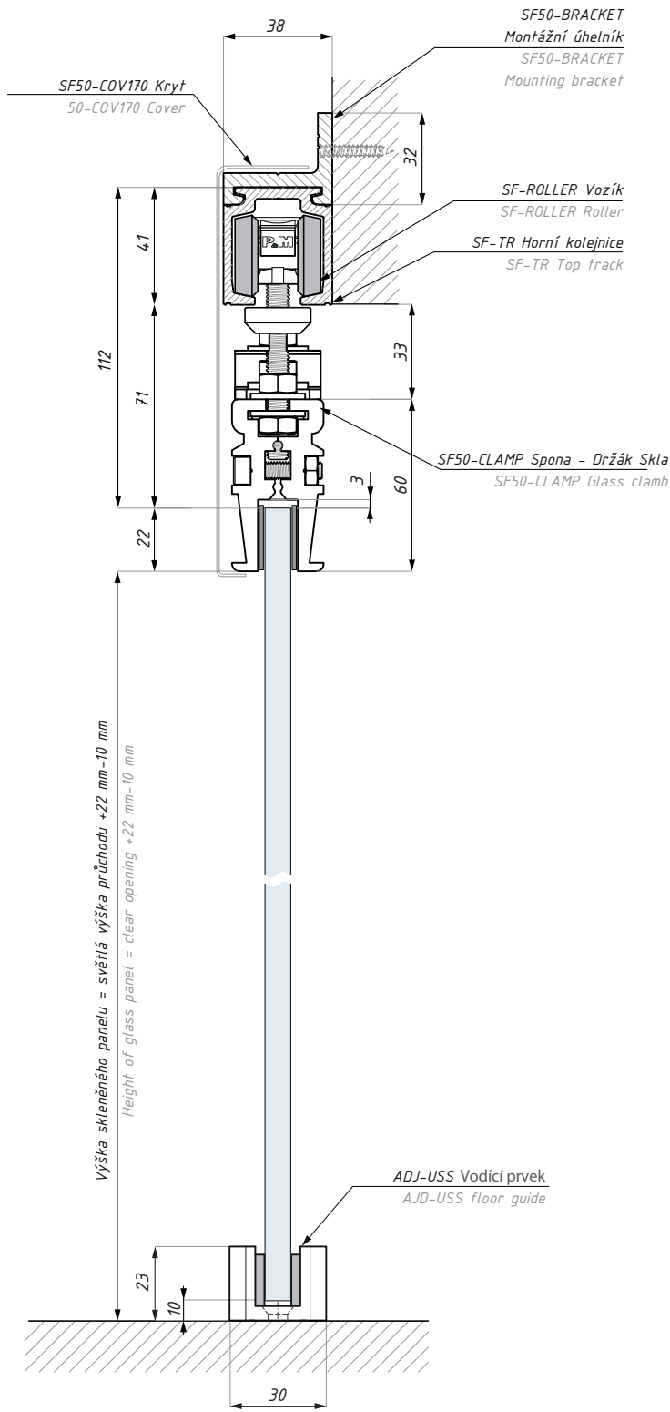
Montáž do stěny Wall instalation
