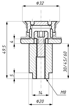
úchyt zapuštěný CSA CSA countersunk routel
