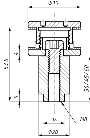
úchyt plochý FHA FHA flathead routel
