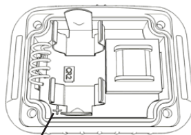
Označení polarity baterie
