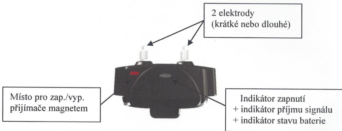
Obr. 1 – Přijímací obojek
