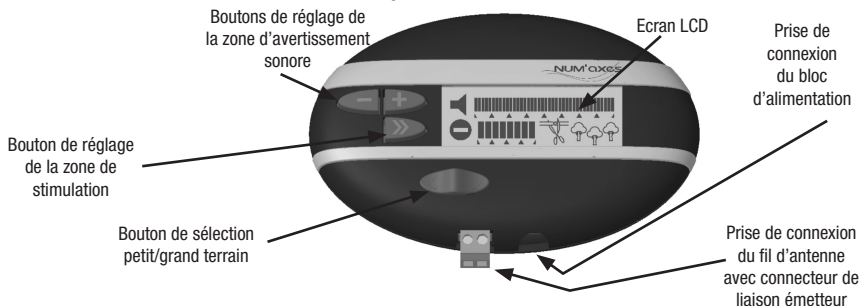
Fig. 1 - Boîtier émetteur
