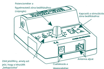
1. ábra: adóegység
