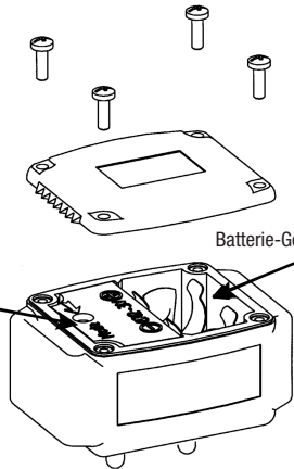
Abb. 3 – Empfänger-Halsband
