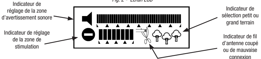
Fig. 2 - Ecran LCD
