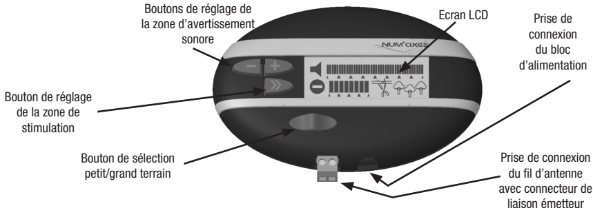
Fig. 1 - Boîtier émetteur
