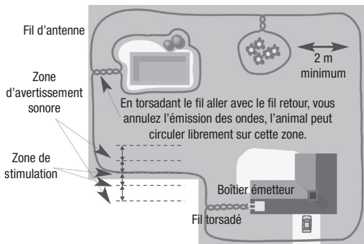
Fig. 4 – Exemple d'installation
