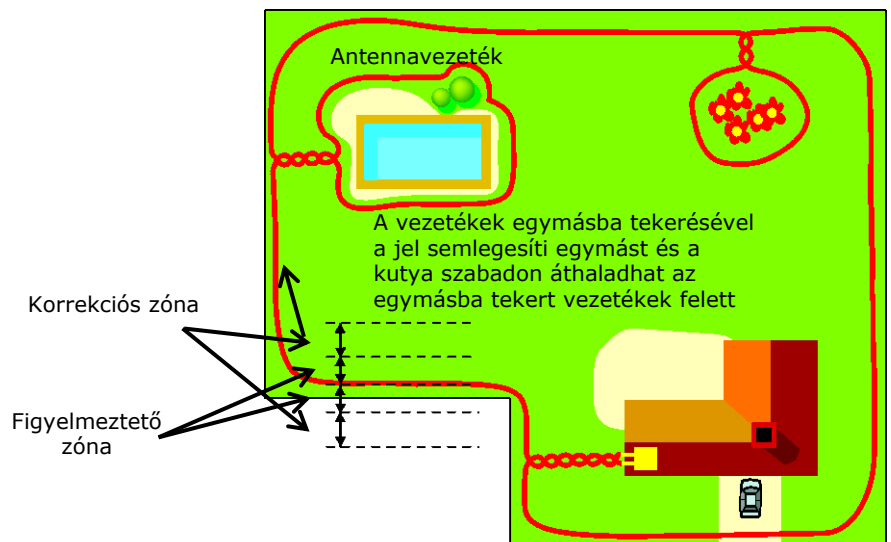
Diagram 3 – Telepítés
