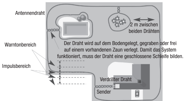
Abb. 3 – Installationsbeispiel
