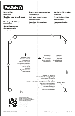
Schneideschablone
