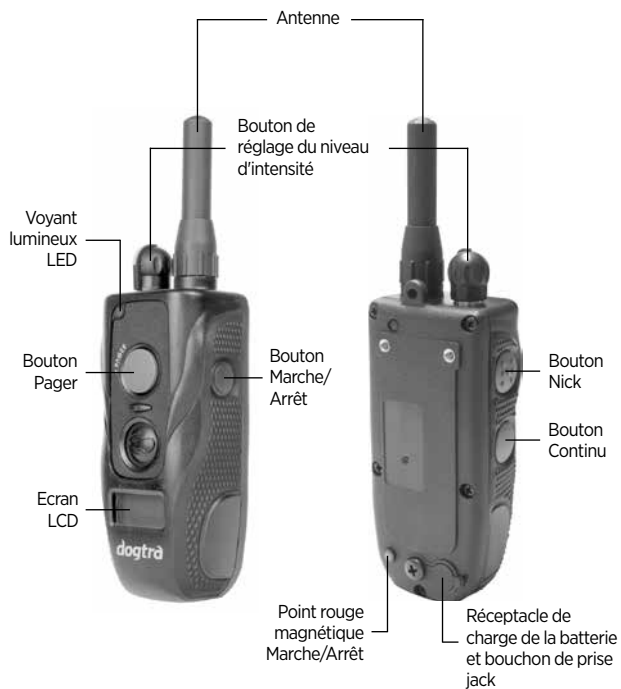
640C Emetteur
