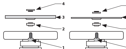
12. ábra. Polírozó sapka (szintetikus pamut), tépőzárás menesztő tányérra, fordulatszám szabályozó sarokcsiszolóhoz
