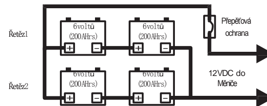
Obr.6, Sériově paralelní zapojení baterie
