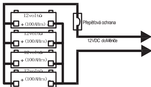
Obr.5, Paralelní zapojení baterií
