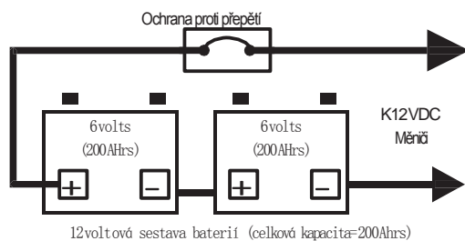
Obr.4, Sériové zapojení baterií
