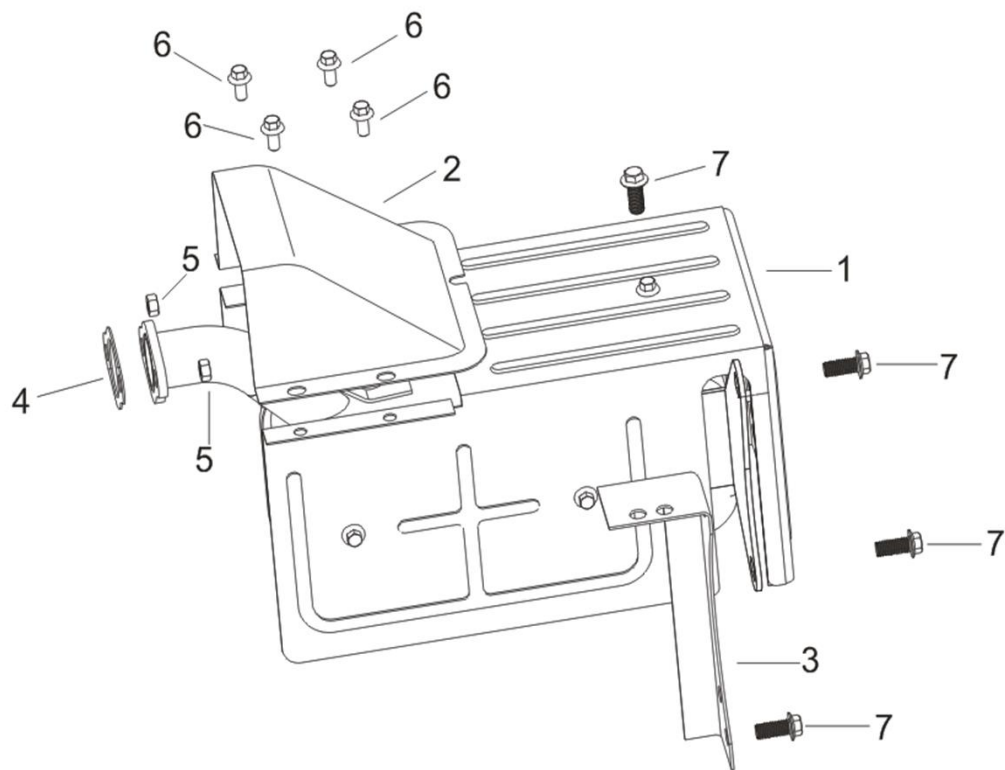
FIG.10 MUFFLER ASSY (F10)
